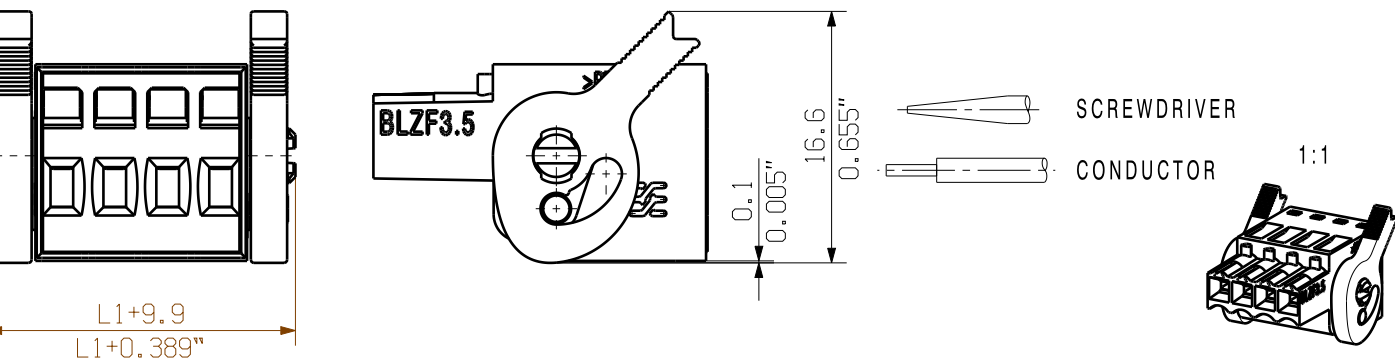
SHOWN:BLZF 3.50/04/180LH
