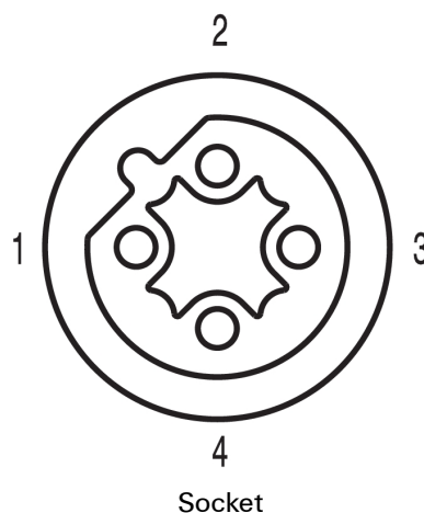
Socket
