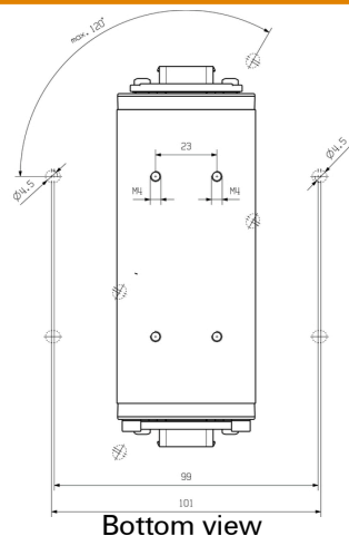
Габаритный чертёж
