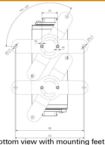
Габаритный чертёж
