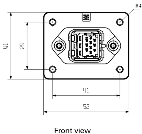
Габаритный чертёж
