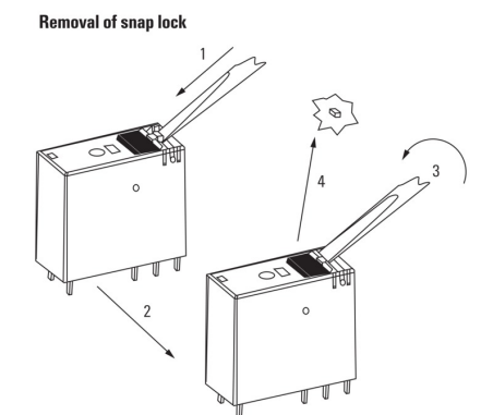
Detailzeichnung Entfernen der Rastsperr der Prüftaste
