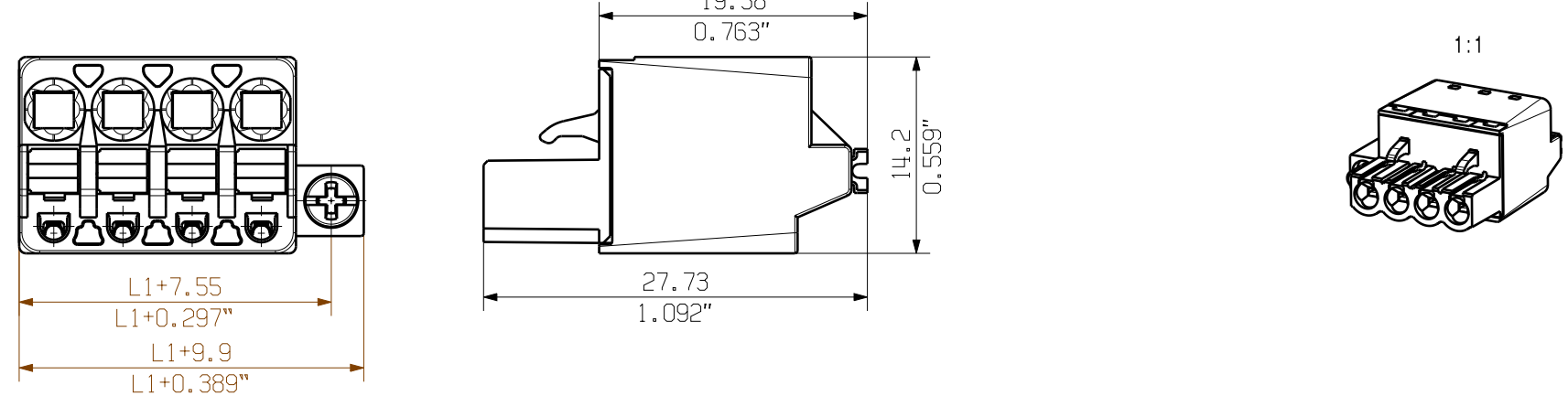
BLF 5.00HC/04/180F SQ SONDERVARIANTE / EINSEITIGER FLANSCH SPECIAL VERSION ONESIDED FLANSH
