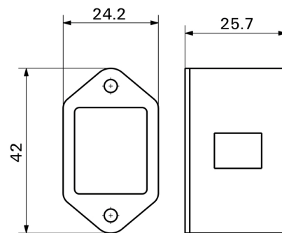
Габаритный чертеж
