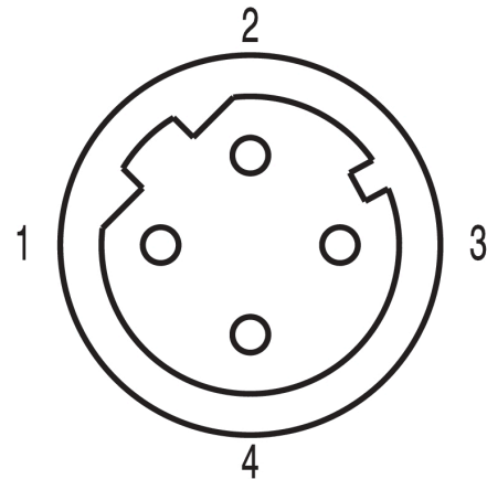
Схема контактов
