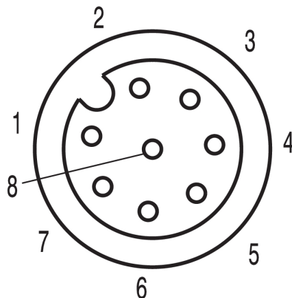
Схема контактов
