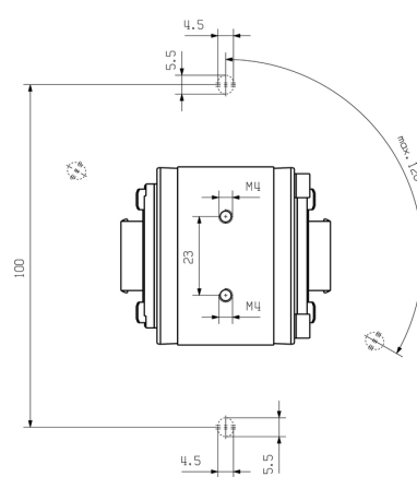
Rysunek wymiarowy
