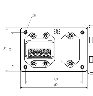
Rysunek wymiarowy
