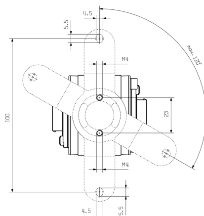
Rysunek wymiarowy
