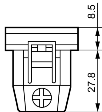
Rysunek wymiarowy
