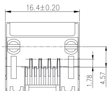
Габаритный чертеж
