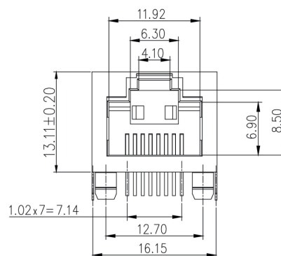
Габаритный чертеж
