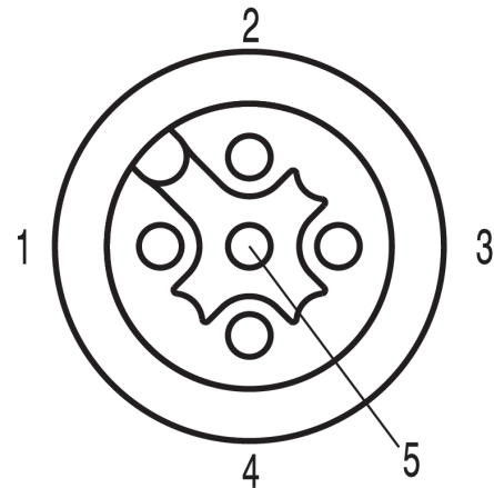
Схема контактов
