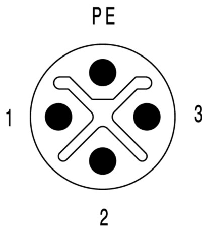
Схема контактов
