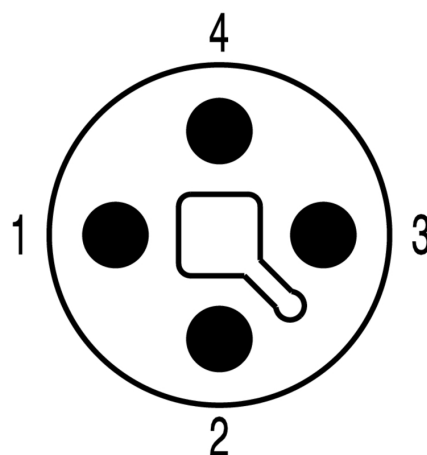
Схема контактов
