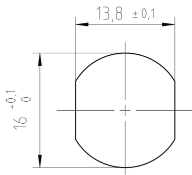
Wycięcie montażowe
