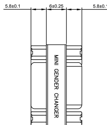
Габаритный чертеж
