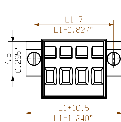
SHOWN:BLZF 3.50/04/180F
