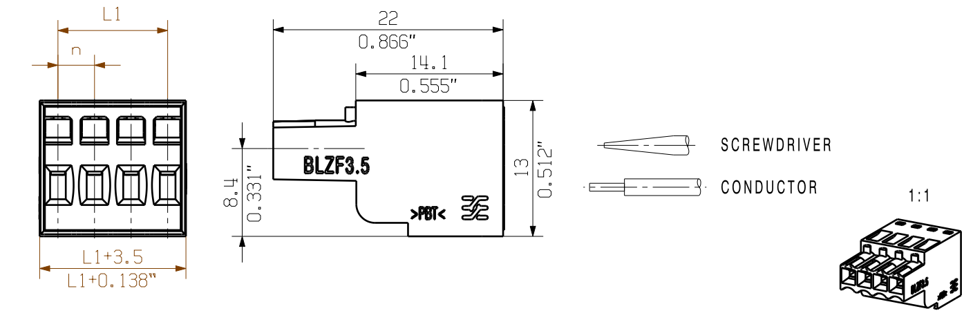
SHOWN:BLZF 3.50/04/180
