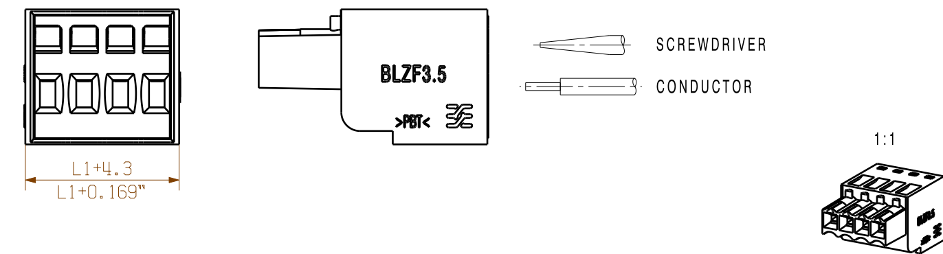
SHOWN:BLZF 3.50/04/180LR
