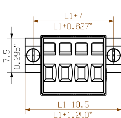
SHOWN:BLZF 3.50/04/180F
