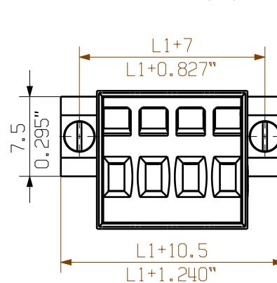
SHOWN:BLZF 3.50/04/180F
