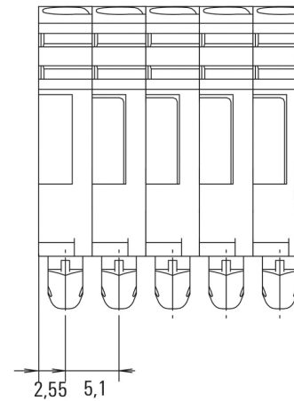
ZDUB 2.5-2/2AN
