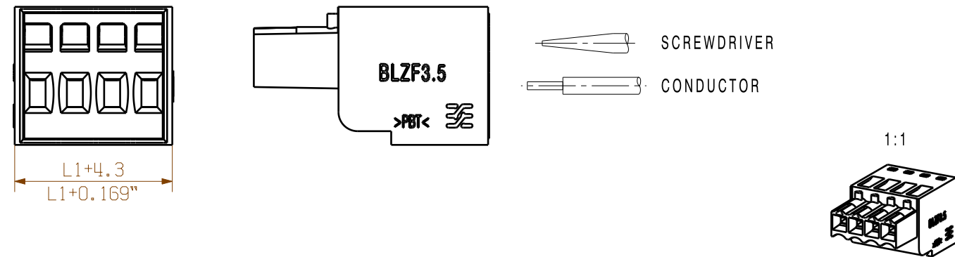
SHOWN:BLZF 3.50/04/180LR
