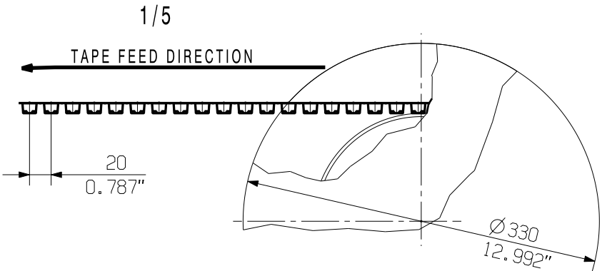
TAPE AND REEL ACCORDING TO IEC 286-3 (EN 60286-3)
