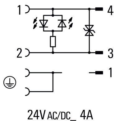
Схема соединений
