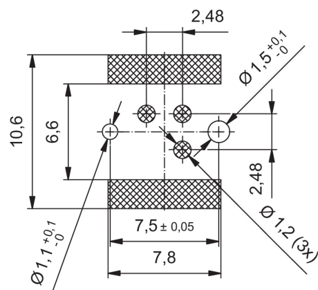
Схема контактов
