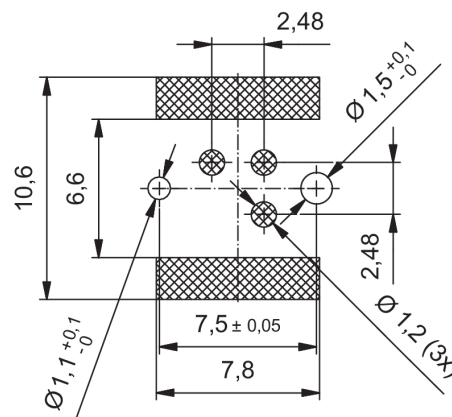
Схема контактов
