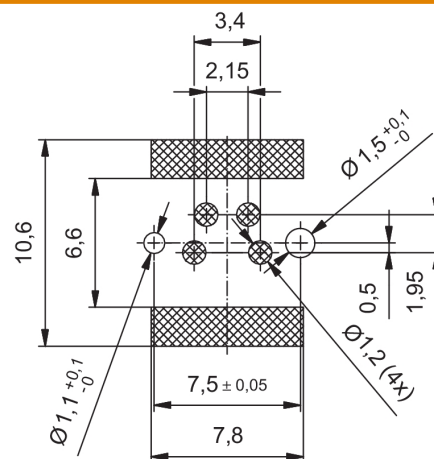
Schemat biegunów
