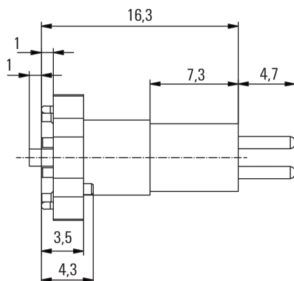
Габаритный чертеж
