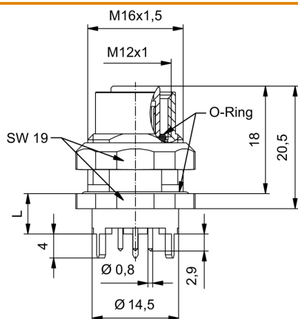
Rysunek wymiarowy
