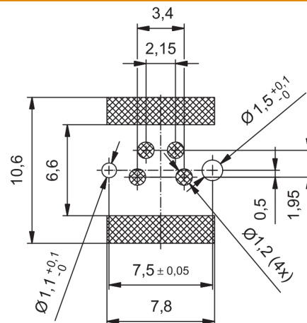
Schemat biegunów
