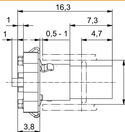
Rysunek wymiarowy
