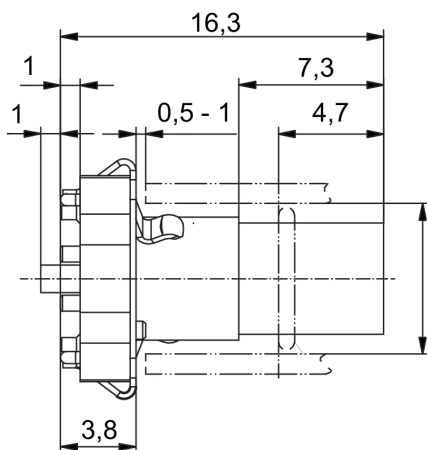
Габаритный чертеж
