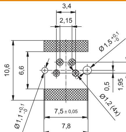
Układ płytek obwodu drukowanego
