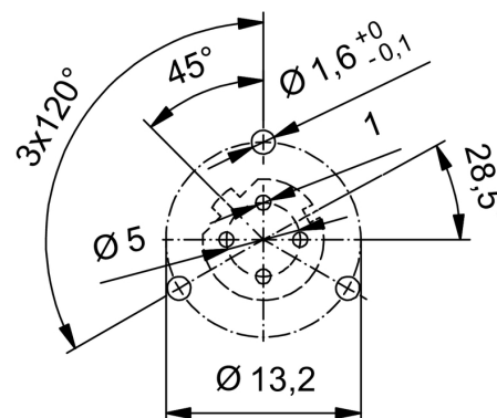
Чертеж РСВ платы
