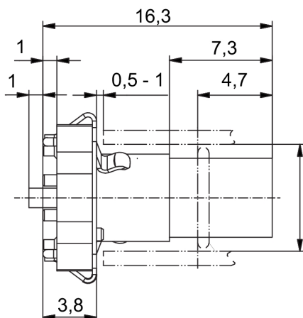
Габаритный чертеж
