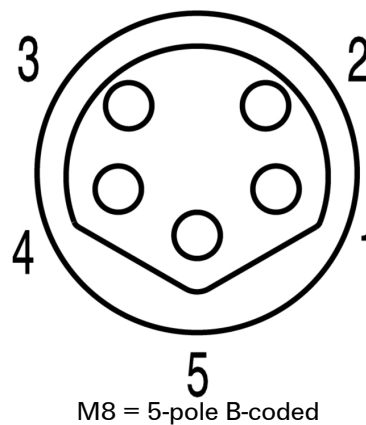
Схема контактов
