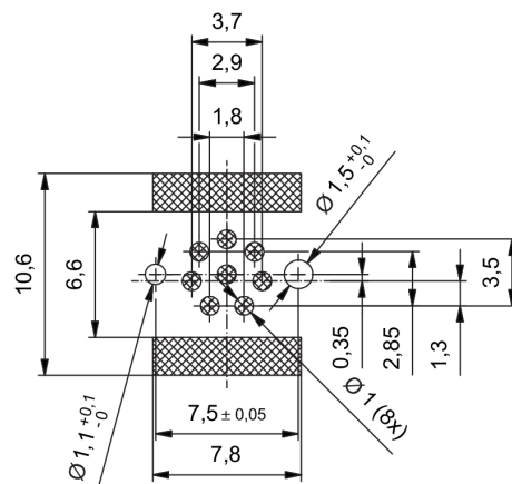
Схема контактов
