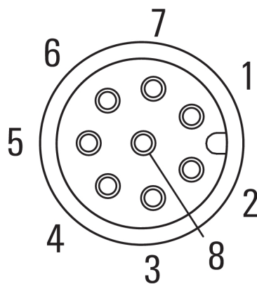
Схема контактов
