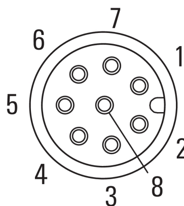
Схема контактов
