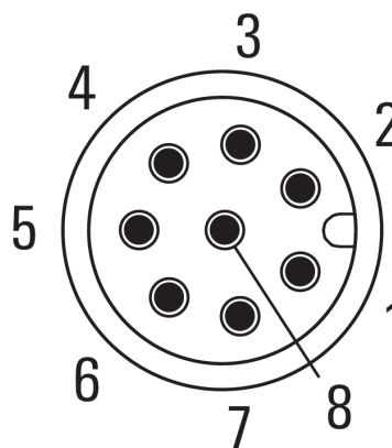
Схема контактов
