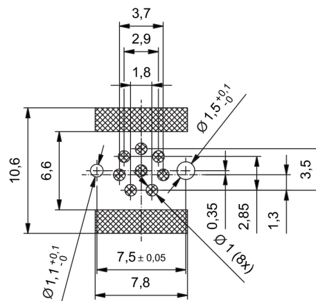
Схема контактов
