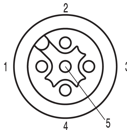
Схема контактов
