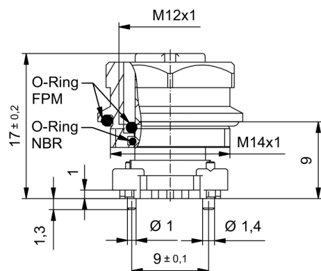
Габаритный чертёж
