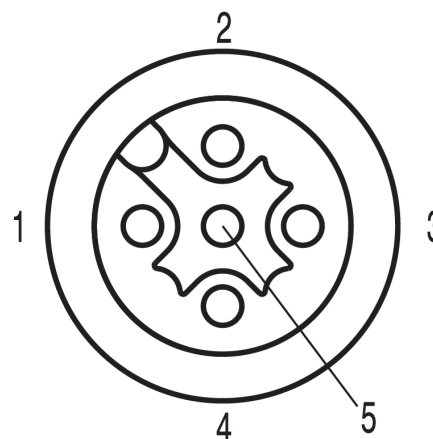
Schemat biegunów
