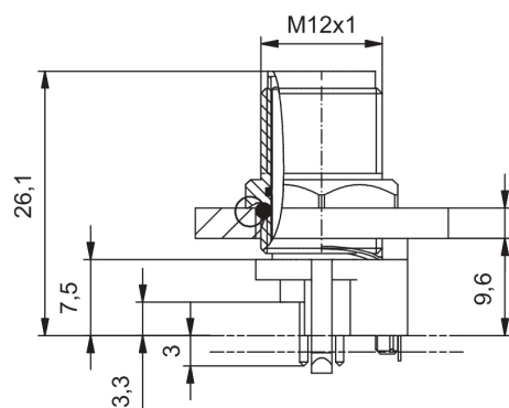
Wycięcie w płycie czołowej
