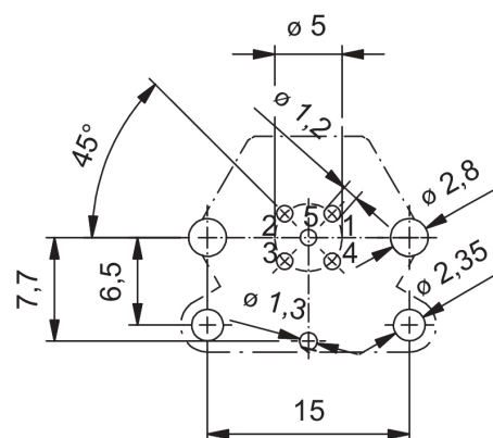
Схема контактов
