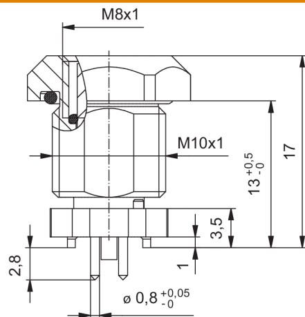
Габаритный чертёж
