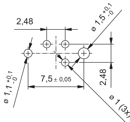
Схема контактов
