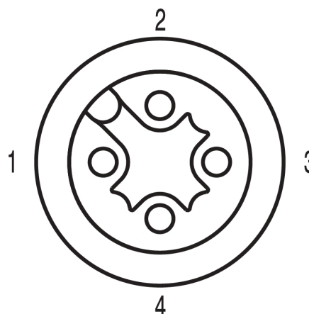
Схема контактов
