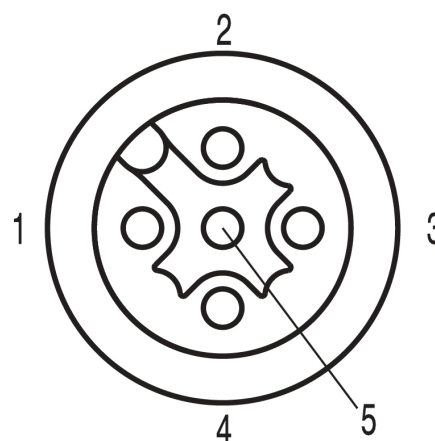
Schemat biegunów
