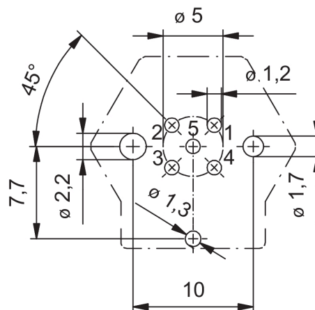
Schemat biegunów
