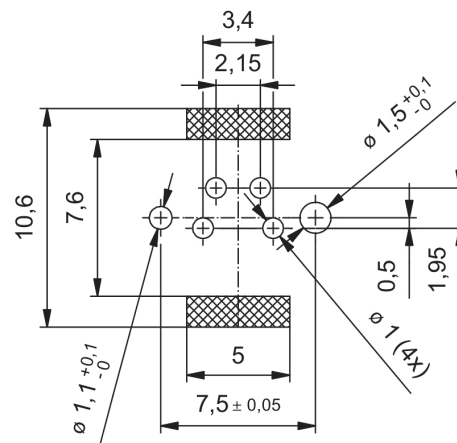
Схема контактов
