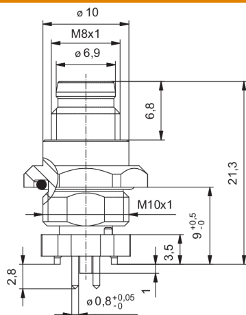
Габаритный чертёж
