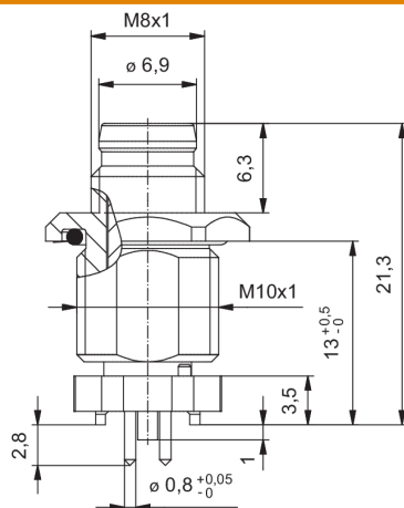
Габаритный чертёж
