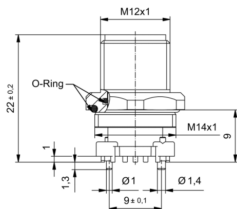
Габаритный чертёж
